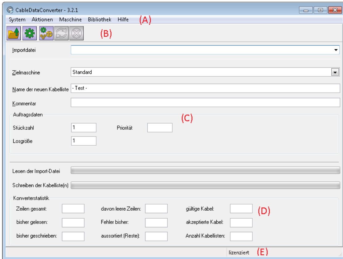
Abbildung 13: Übersicht - CableDataConverter Hauptfenster
