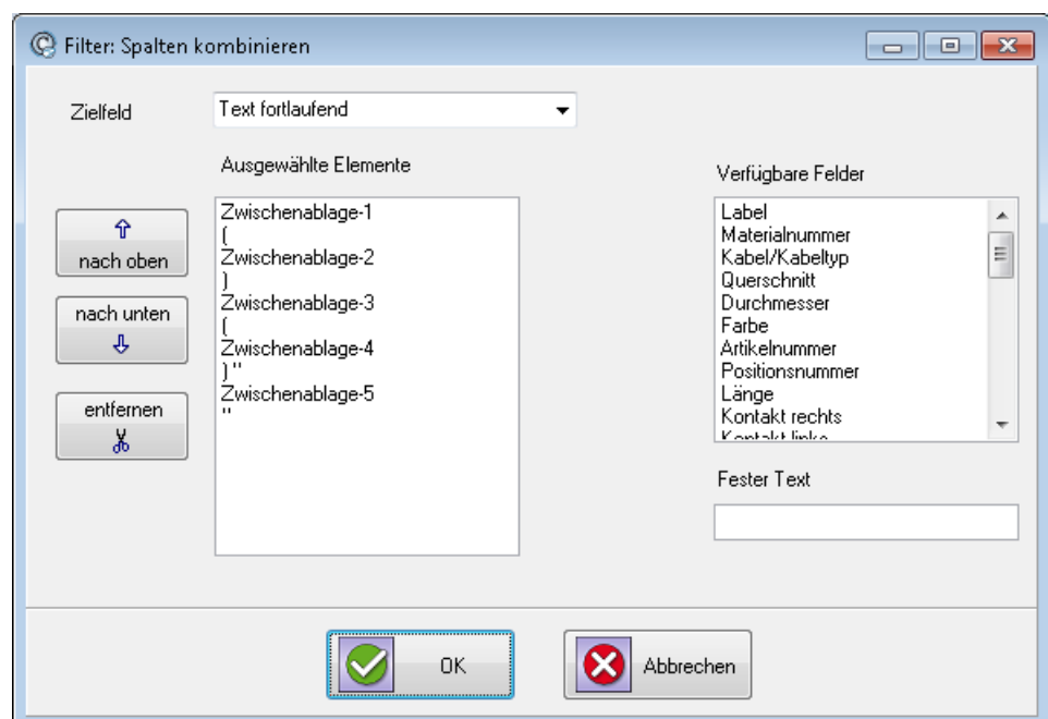
Abbildung 23: Beispiel: Spalten kombinieren mit Zwischenablage
