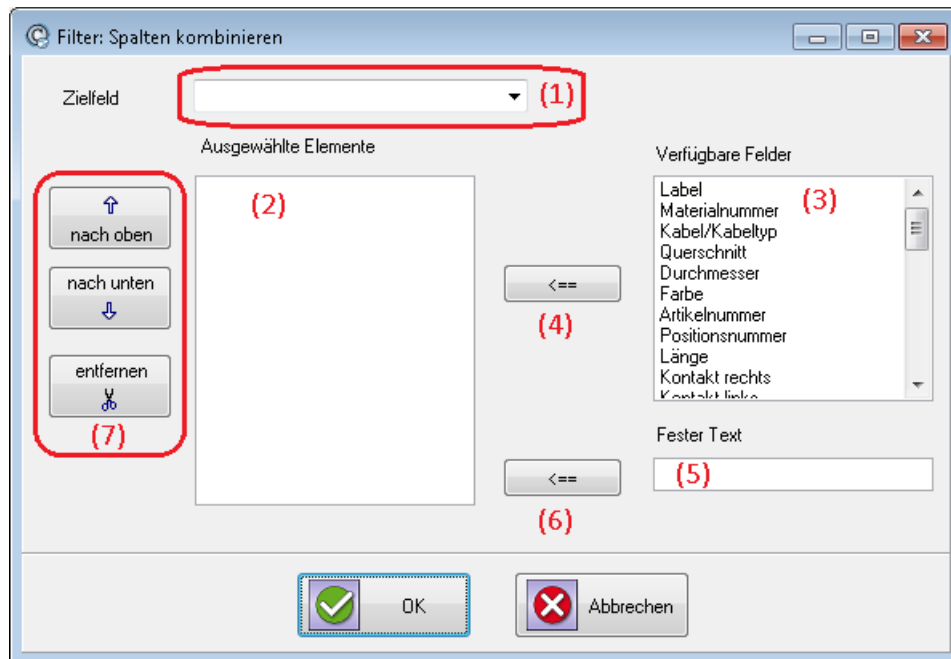
Abbildung 21: Filtereinstellung: Kombination mehrerer Spalten
