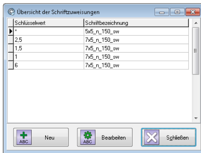
Abbildung 38: Übersicht - Schriftzuweisungen
