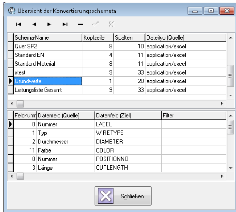
Abbildung 36: Übersicht - Konvertierungsschemata
