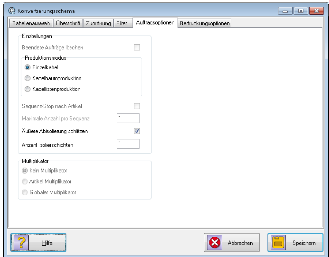
Abbildung 24: Konvertierungsschema - Auftragsoptionen
