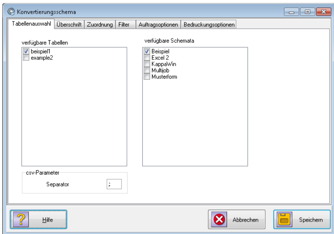
Abbildung 15: Konvertierungsschema - Tabellenauswahl
