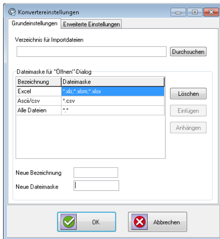
Abbildung 33: Konvertereinstellungen
