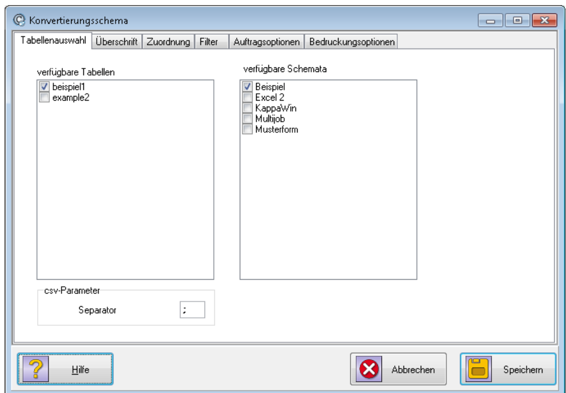
Abbildung 14: Übersicht - Konvertierungsschema
