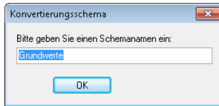
Abbildung 28: Eingabe - Schemaname
