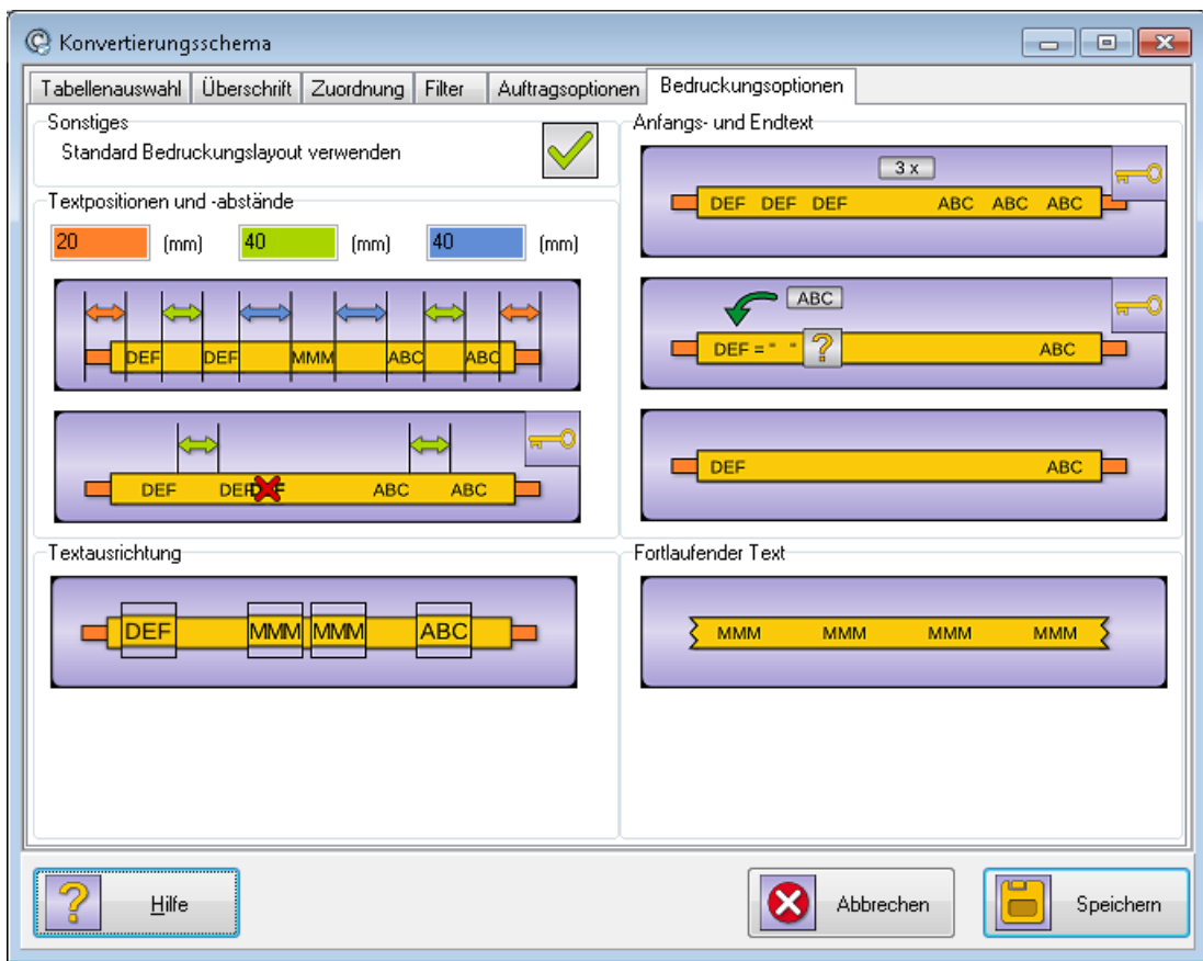
Abbildung 27: Konvertierungsschema - Bedruckungsoptionen
