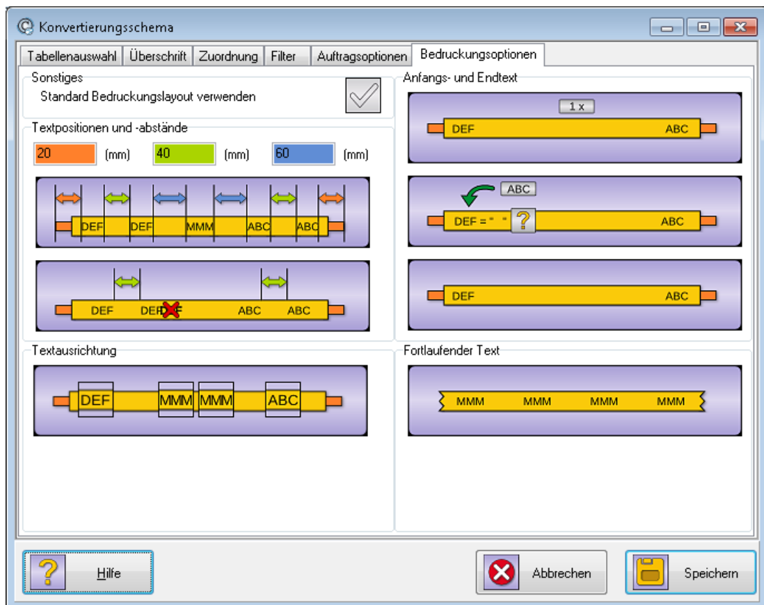
Abbildung 25: Konvertierungsschema - Bedruckungsoptionen
