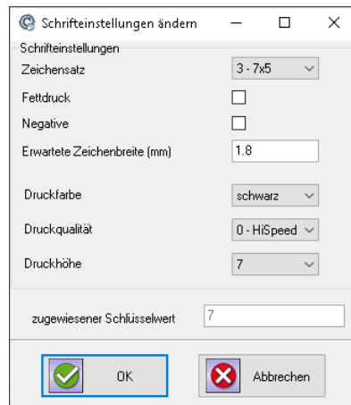
Abbildung 48: Schriftzuweisung
